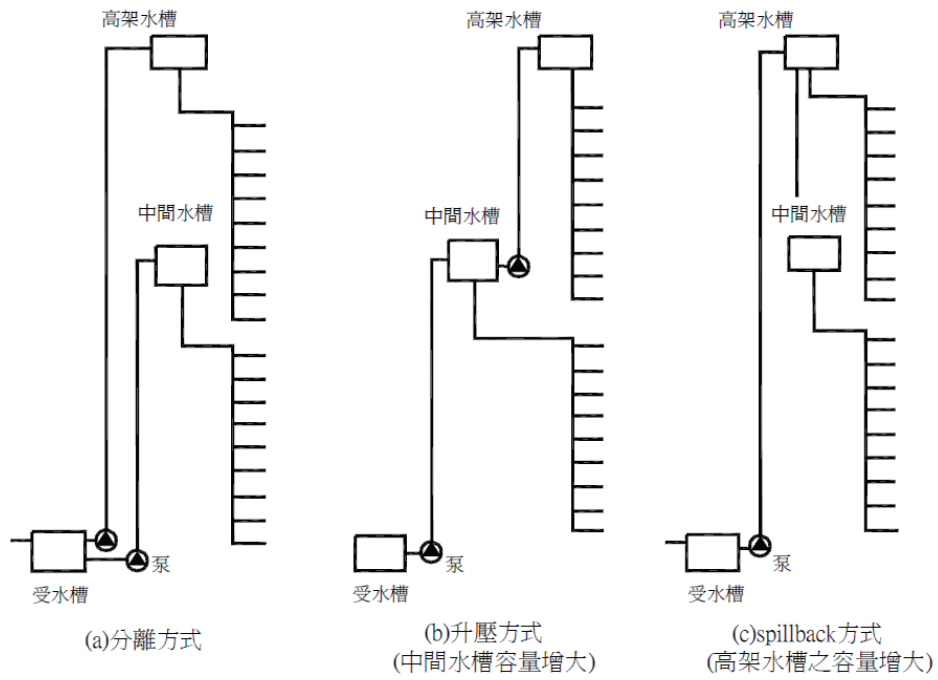
圖3-8 利用中間水槽之給水配管分區示意圖
