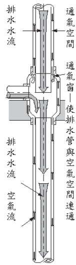
圖4-7 排水通氣二層管方式
