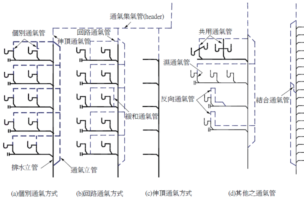
圖4-4 通氣方式與通氣管
