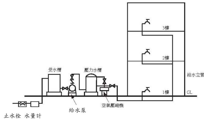
圖3-2 壓力水槽給水系統圖
