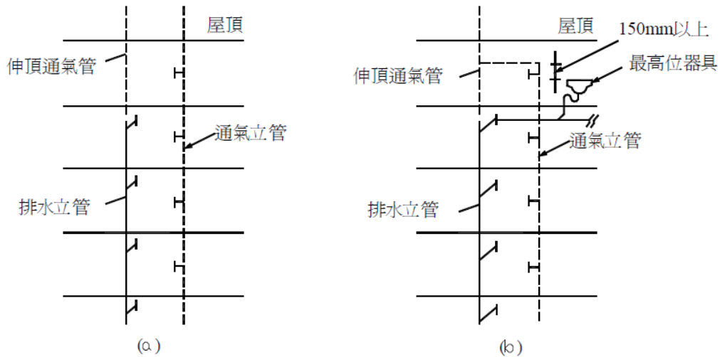
圖4-11 通氣立管上部處理
