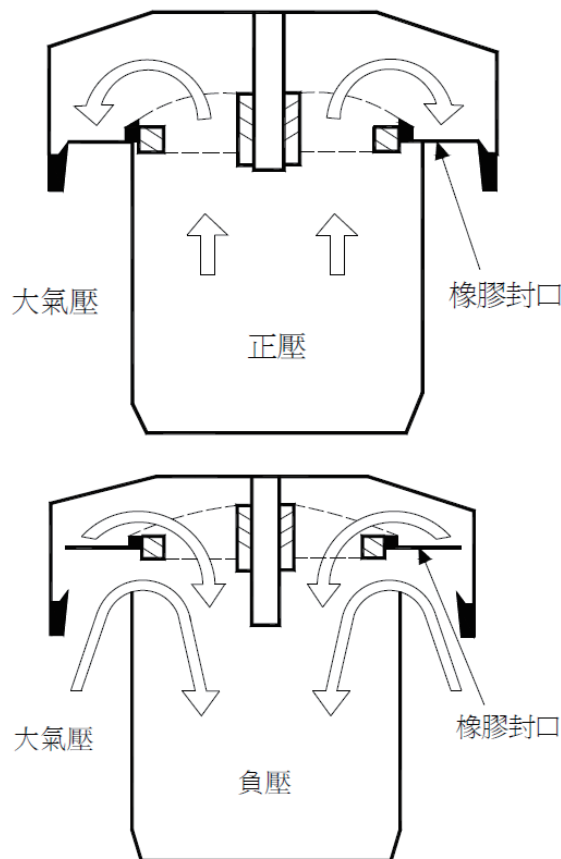
圖4-16吸氣閥構造圖例
