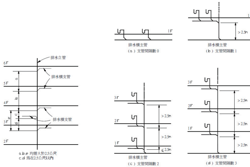
圖4-3 排水分支間隔計算圖示
