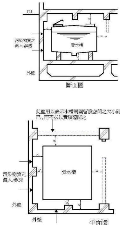
說明：a、a' b、c 表示為易於進行維護檢查所需留設之距離 (a,b,c ≥ 60cm) (a' ≥ 45cm)
