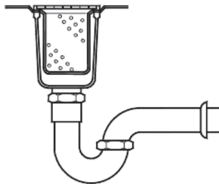
圖4-21 毛髮截留器參考圖例
