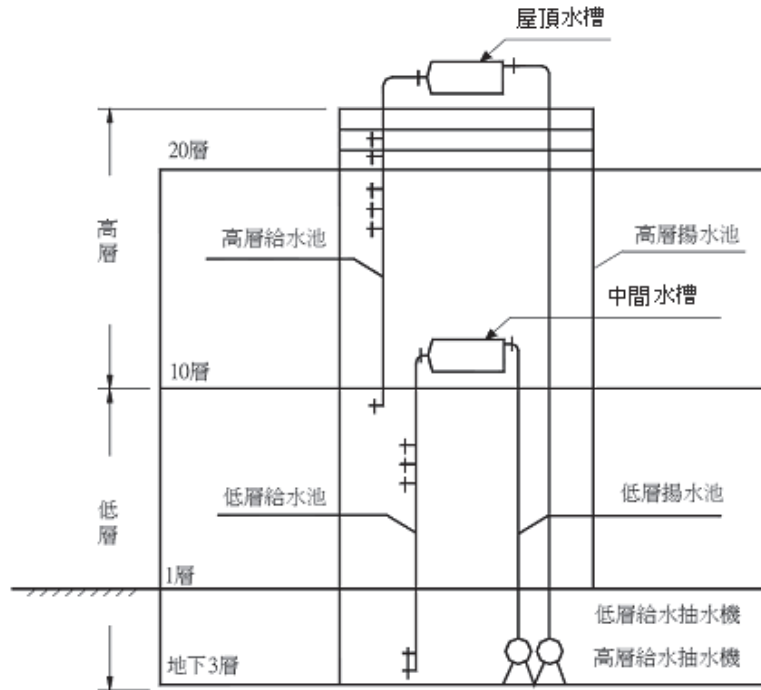
圖3-6 間接給水設置中間水槽示意圖
