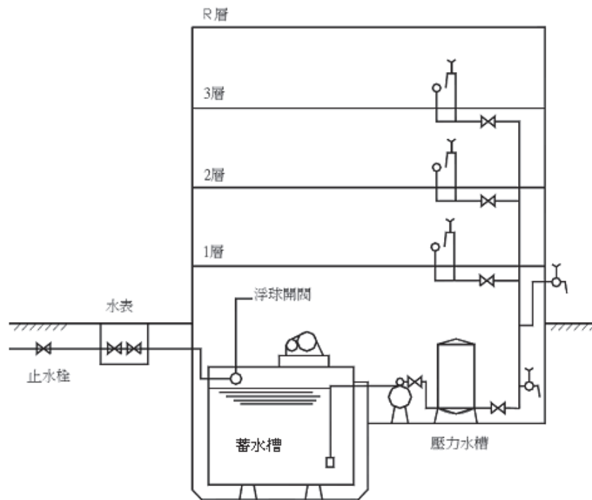
圖3-7 間接給水直接加壓方式示意圖
