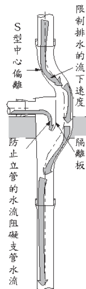
圖4-6 抑制排水流下速度方式
