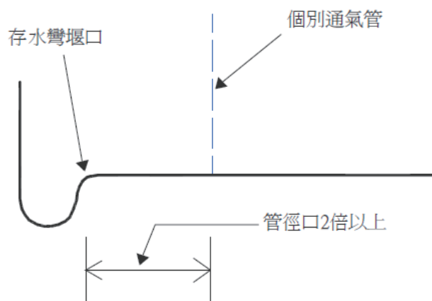
圖4-13 存水彎堰口與通氣管的距離
