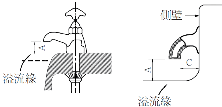
圖3-10 飲用水槽之出水口空間(A)
