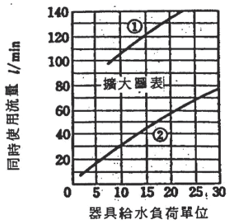
圖 A-4 器具給水負荷單位同時使用流量線圖
