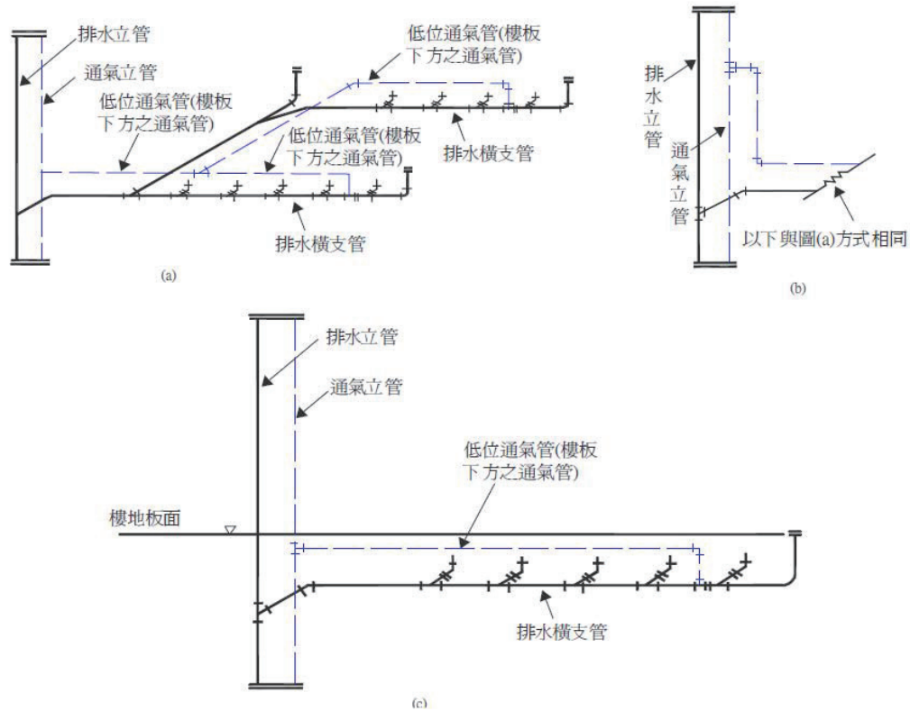
圖4-10 通氣管安裝之錯誤設計圖例
