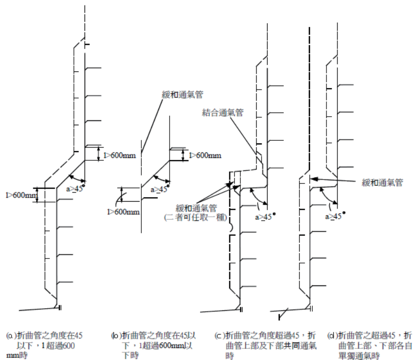
圖4-2 立管、折曲管與排水橫主管之關係
