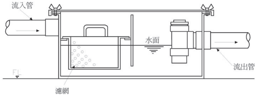
圖4-23 固體物截留器參考圖例
