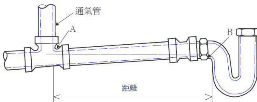
圖4-13 存水彎堰口與通氣管的距離
