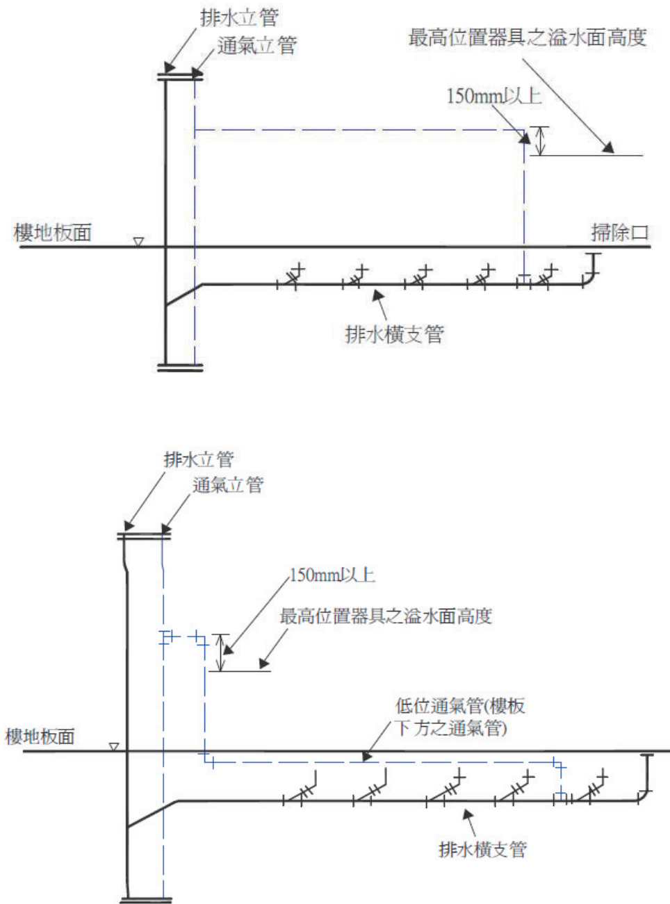
圖4-9 有條件之低位通氣管安裝圖例
