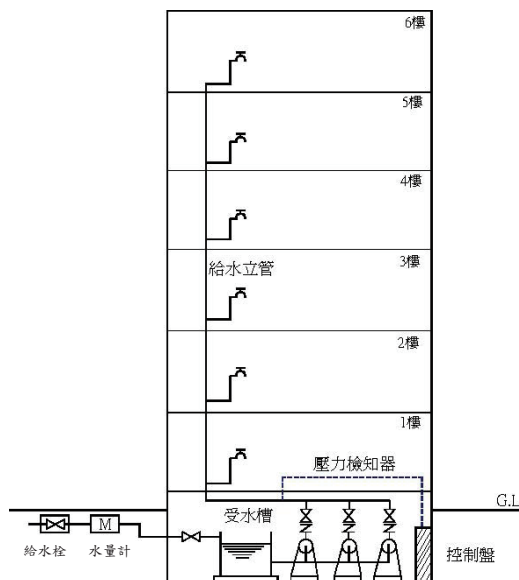
圖3-4 加壓泵給水系統圖
