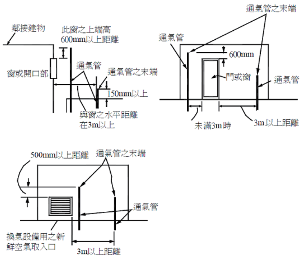
圖4-12 通氣管末端開口部之位置
