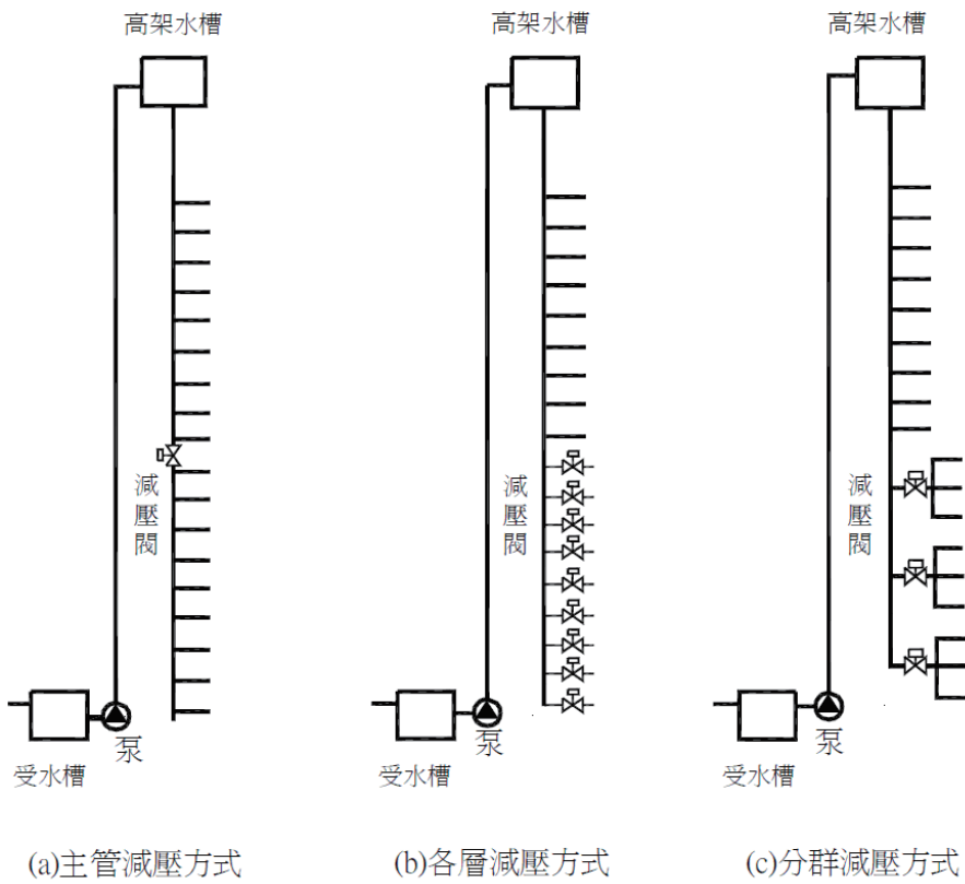
圖3-9 利用減壓閥之給水配管分區示意圖
