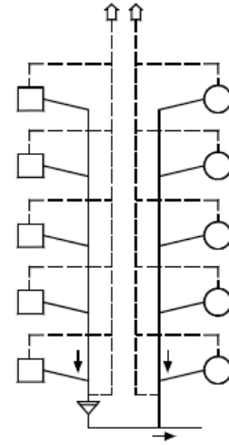
b. 全通氣二立管方式
