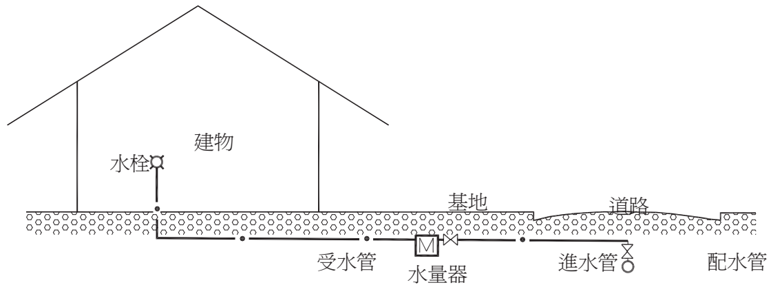
圖3-1 直接給水系統圖
