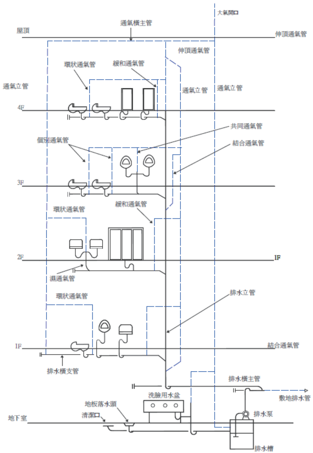
圖4-8 排水通氣系統圖
