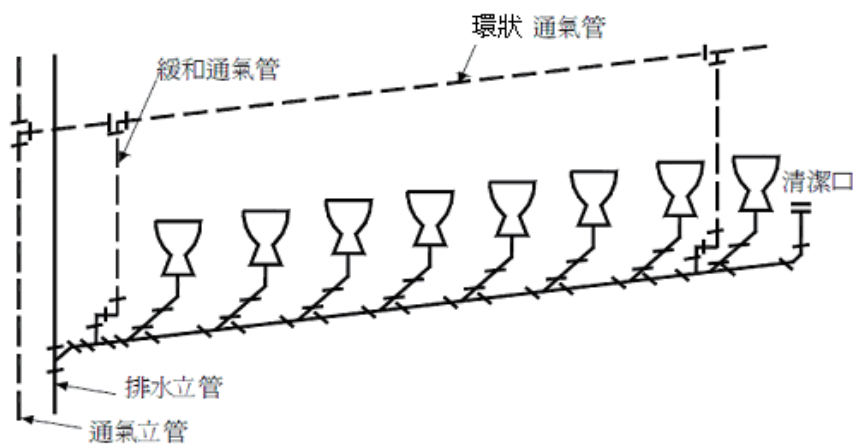
圖4-15 環狀通氣管與緩和通氣管安裝圖例
