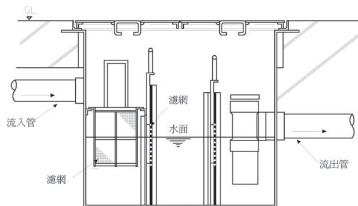
圖4-22 纖維毛髮截留器參考圖例
